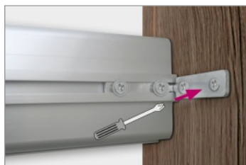
montáž profilu S157 ku korpusu
