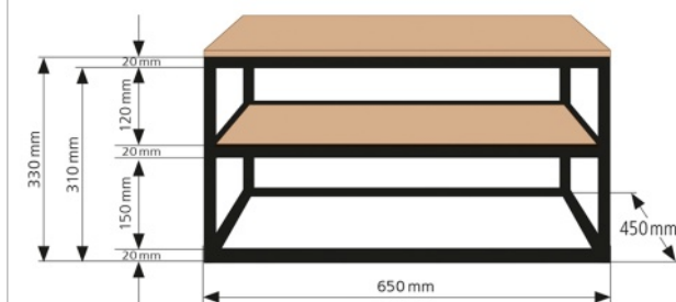
Konferenčný stolík - Výkres pre cenovú ponuku
