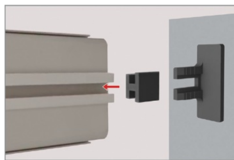
umiestnenie protikusu k úchytu
