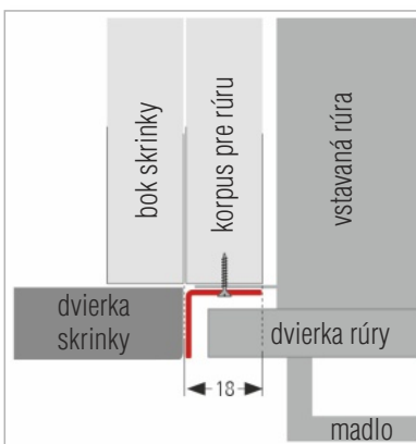
Umiestnenie bočnej ochrannej lišty MT/bočná (ľavá strana, pohľad zhora)
