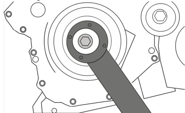
Kurbelwellen-Riemenscheiben- Gegenhalteschlüssel OEM T10355
