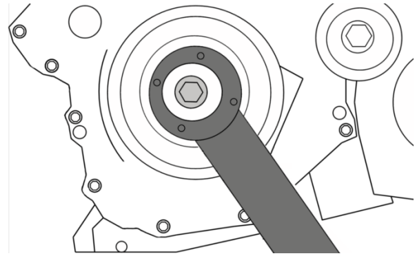
Clé de maintien de poulie de vilebrequin, à utiliser comme OEM T10355
