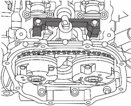
Nockenwellen-Fixierung, zu verwenden wie OEM T40070
