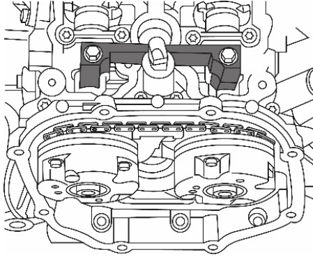
Blocage d'arbre à cames, à utiliser comme OEM T40070
