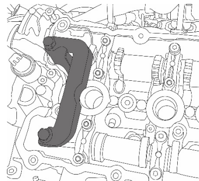
Blocage d'arbre à cames, à utiliser comme OEM T40133
