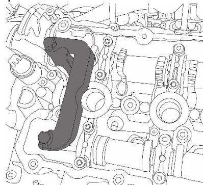
Fijación del árbol de levas, para usar como OEM T40133
