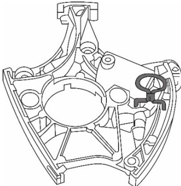
Bloqueo de tensores de cadena, para usar como OEM T40071
