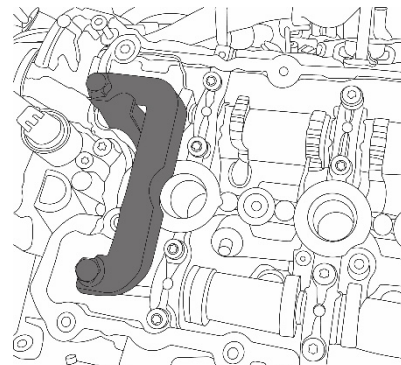
Nockenwellen-Fixierung, zu verwenden wie OEM T40133
