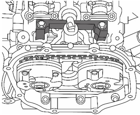
Fijación del árbol de levas, para usar como OEM T40070
