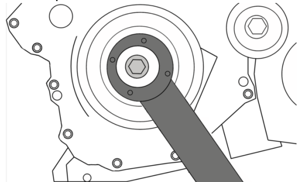
Llaves de sujeción de la polea del cigüeñal, para usar como OEM T10355
